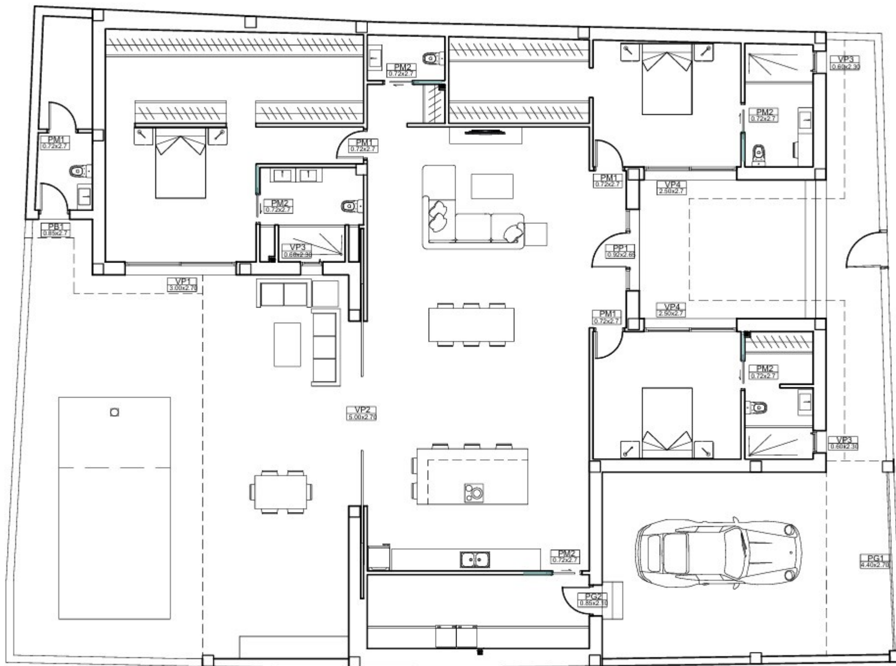
PLANTA BAJA
